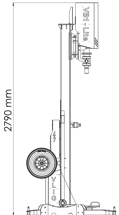
LEFT SIDE
